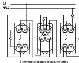
2 interruptores paralelos iluminados
