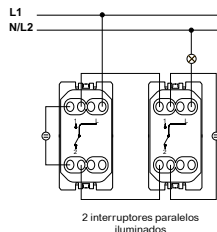
2 interruptores paralelos iluminados
