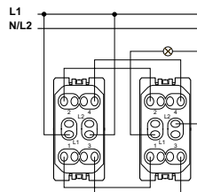
Interruptor bipolar paralelo
